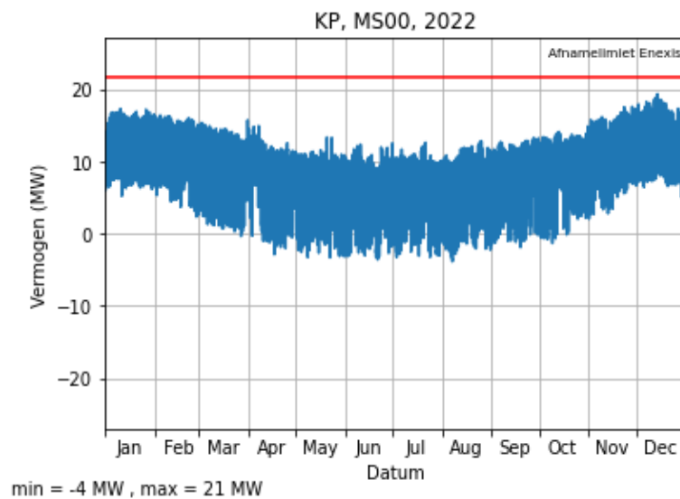
Figuur 2. Gemeten transportbelasting op HS/MS-station Kampen blok 0 in 2022. Een positieve waarde representeert afname van het hoogspanningsnet. De aanwezige transportcapaciteit voor afname bedraagt 22 MW.
