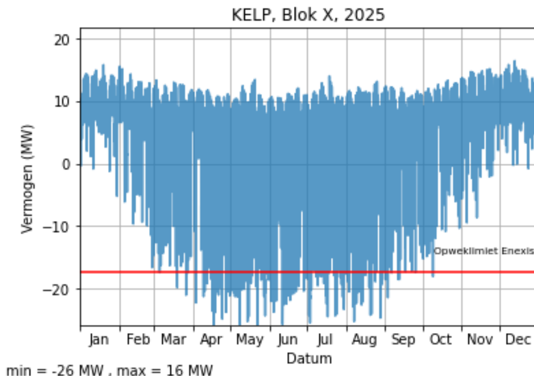
Figuur 3. Verwachte transportschaarste op station Kelpen in het laatste jaar van de congestie.
