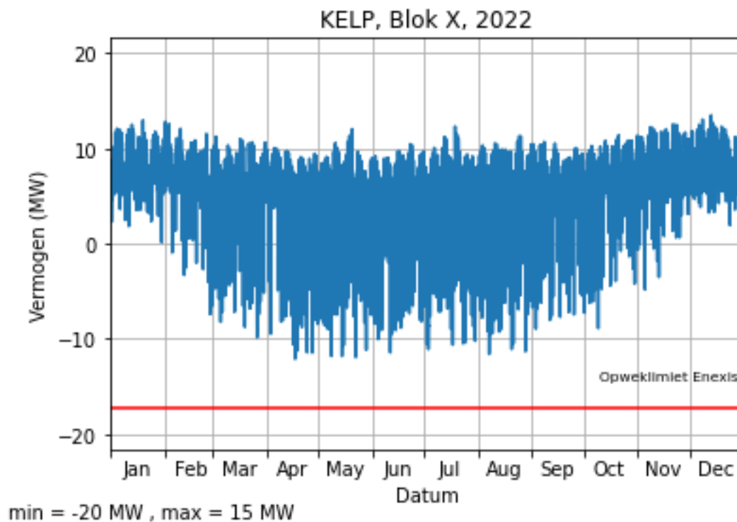
Figuur 2. Gemeten transportbelasting op station Kelpen in 2022. Een negatieve waarde representeert terug levering aan het HS-net. De huidige, aanwezige transportcapaciteit voor teruglevering bedraagt 17,0 MW.
