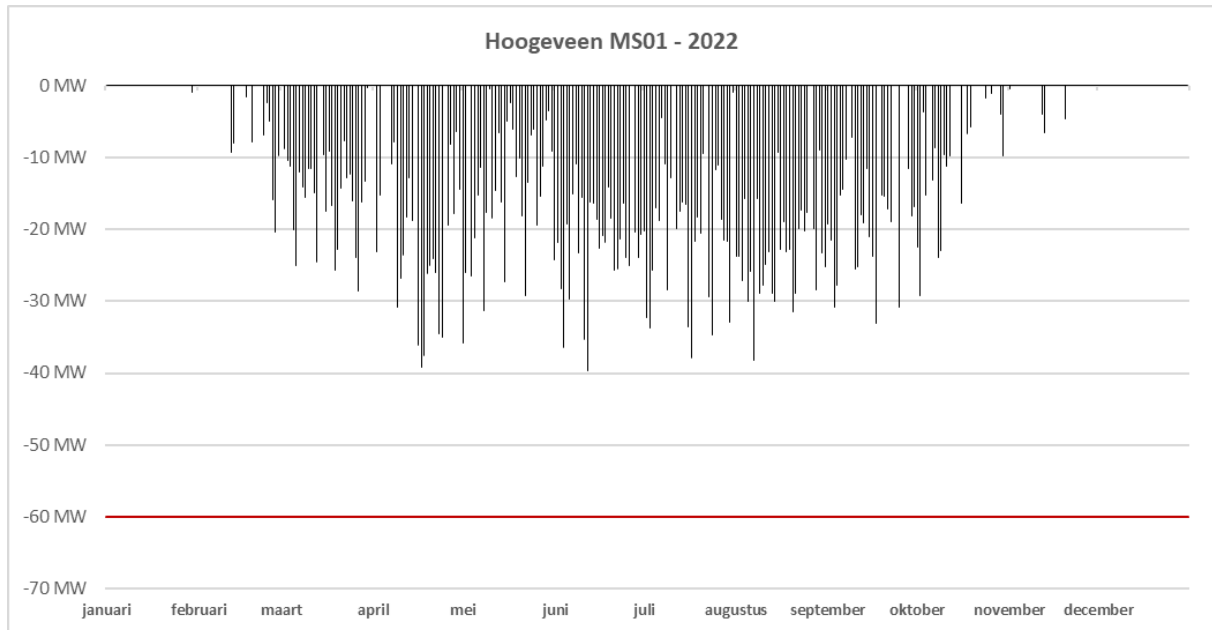
Figuur 2. Gemeten transportbelasting op station Hoogeveen MS01 in 2022. Een negatieve waarde representeert invoeding in het hoogspanningsnet. De huidige, aanwezige transportcapaciteit voor invoeding bedraagt 60,0 MW.
