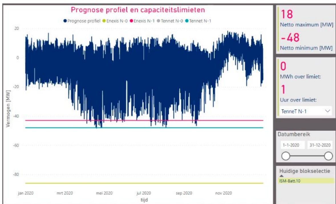
Figuur 2 - Belasting in 2022 (gemeten waarden 2020 + alle reeds in opdracht gegeven aansluitingen)
