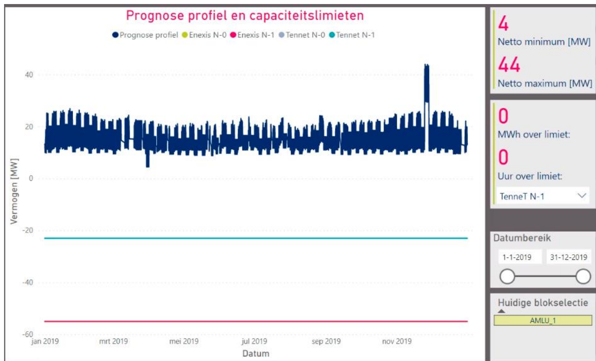
Figuur 1 – Actuele belasting
