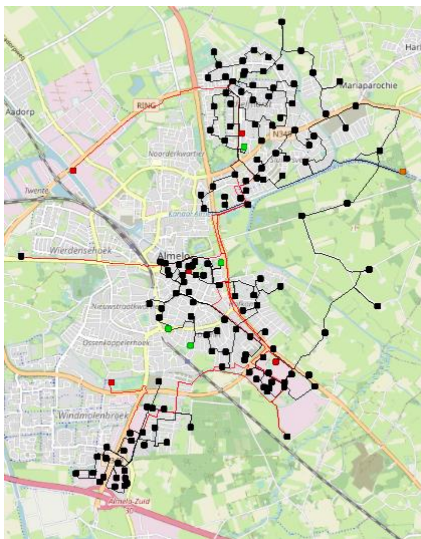
Figuur 2b: Geografisch overzicht verzorgingsgebied HS/MS station Almelo Urenco (Coteq)
