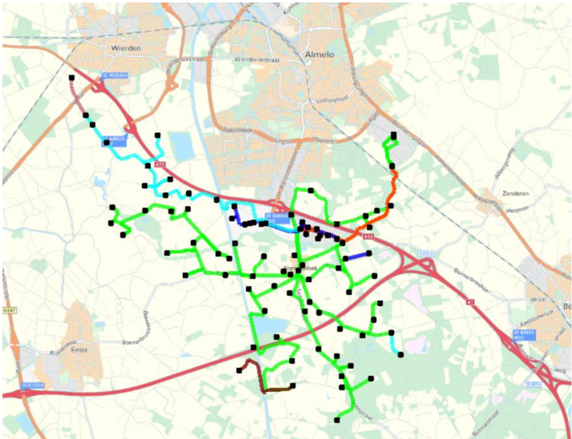
Figuur 1a: Geografisch overzicht verzorgingsgebied HS/MS station Almelo Urenco (Enexis)
