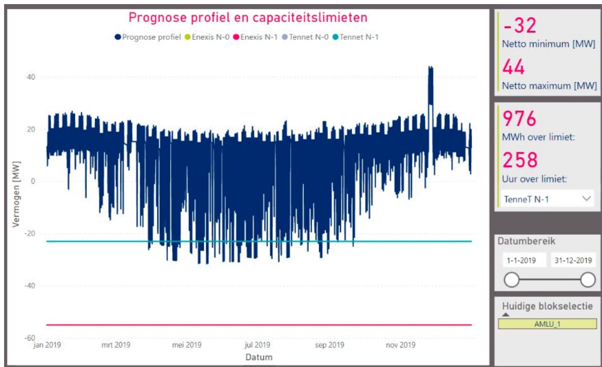
Figuur 4 - Verwachte belasting 2023 en verder (meetwaardes 2019, alle opdrachten en bekende initiatieven)
