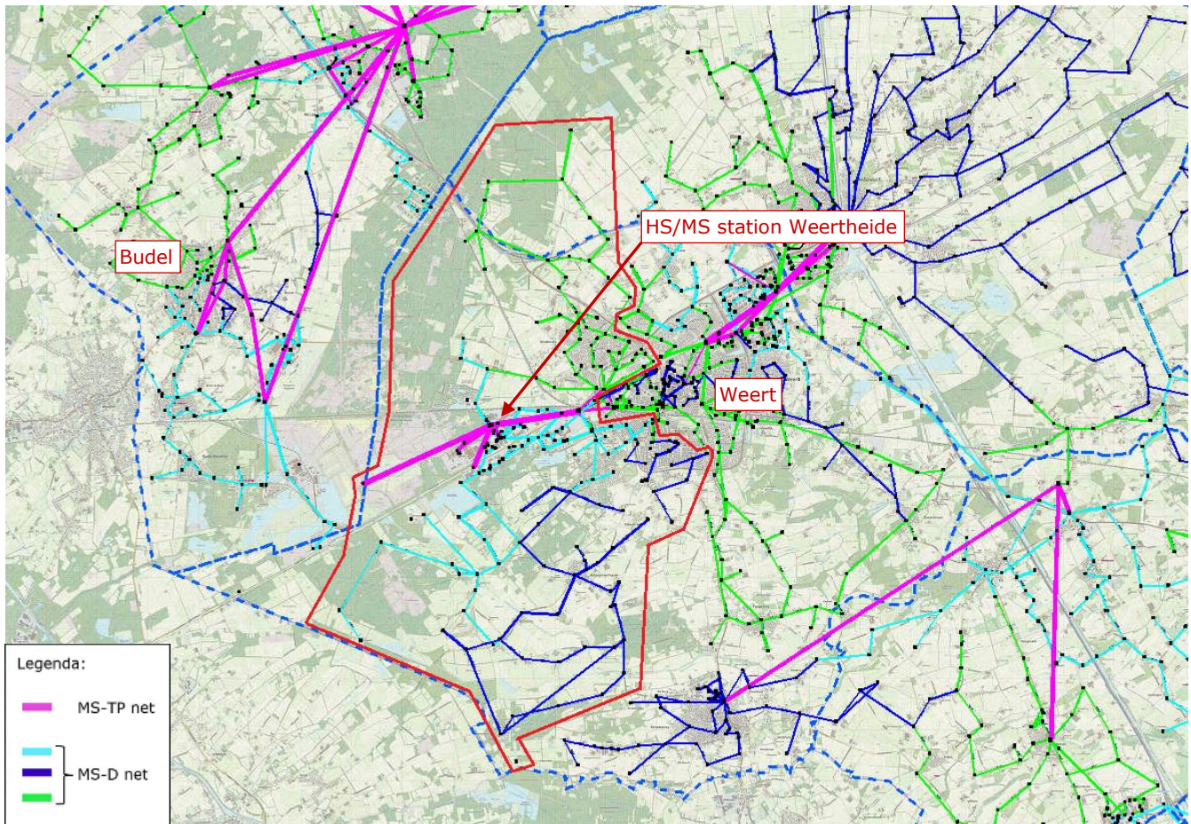
Figuur 1: Geografisch overzicht verzorgingsgebied HS/MS station Weertheide
