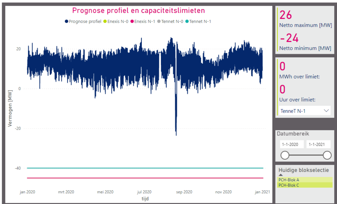
Figuur 3 – Actuele belasting (dip van -24 MW dient te worden genegeerd)
