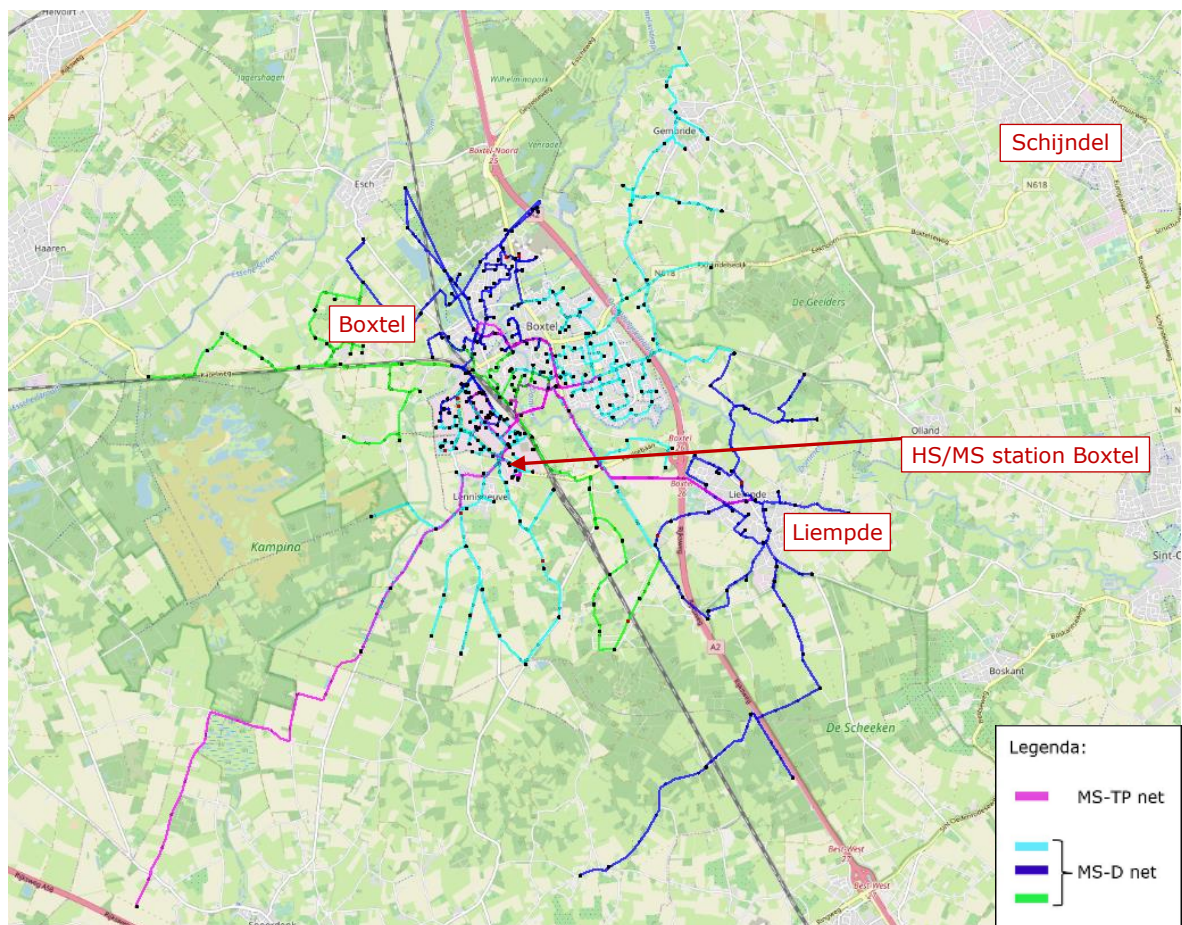
Figuur 1: Geografisch overzicht verzorgingsgebied HS/MS station Boxtel
