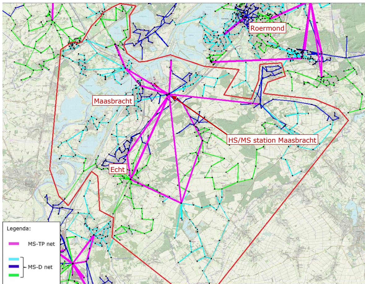
Figuur 1: Geografisch overzicht verzorgingsgebied HS/MS station Maasbracht
