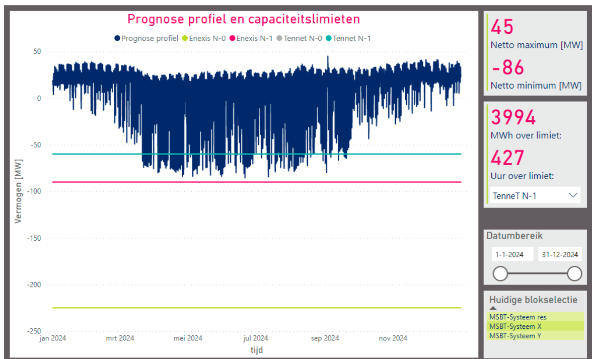
Figuur 5 - Verwachte belasting 2024 en verder (meetwaarden 2020, alle opdrachten en bekende initiatieven)
