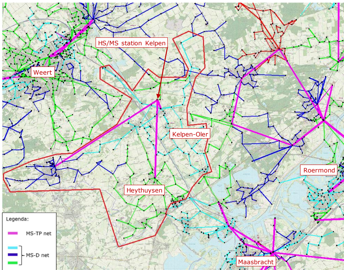
Figuur 1: Geografisch overzicht verzorgingsgebied HS/MS station Kelpen
