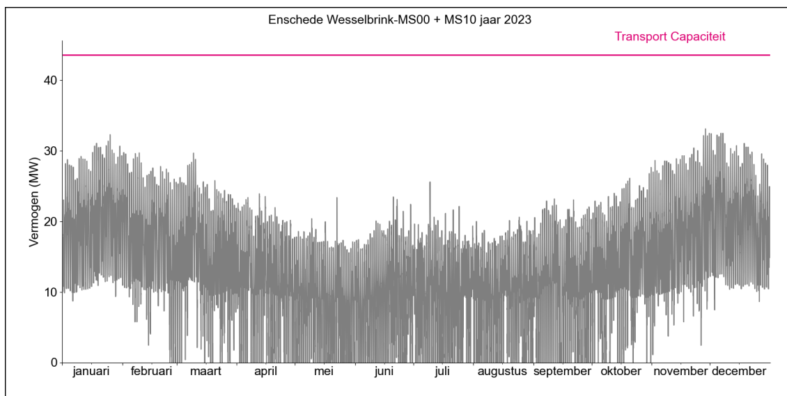
Figuur 2. Gerealiseerde transportbelasting voor afname op HS/MS-station Enschede Wesselerbrink MS00 + MS10 in 2023.
