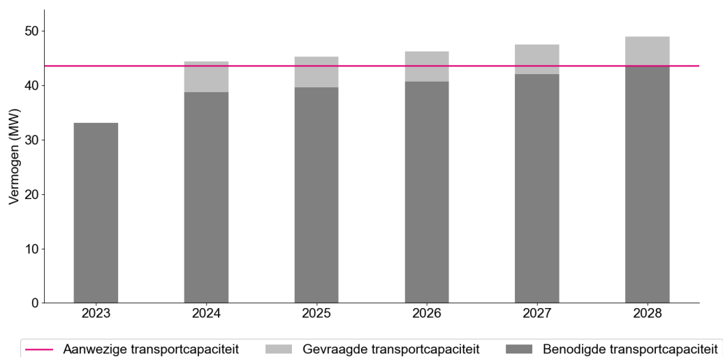
Benodigde en gevraagde transportcapaciteit Afname ESDW-MS00 + MS10
