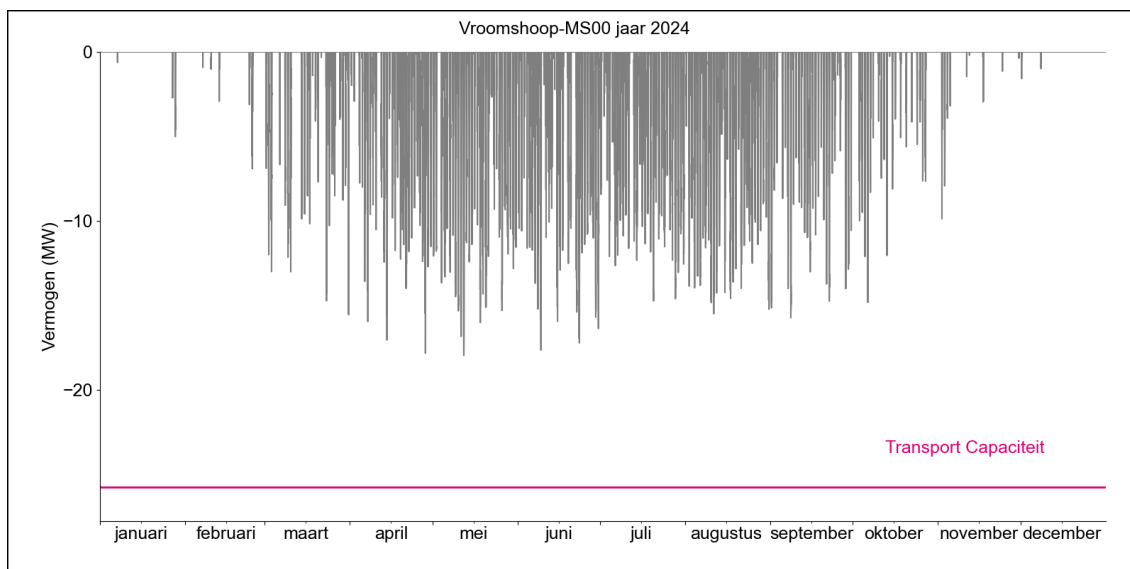
Figuur 2. Gerealiseerde transportbelasting voor invoeding op HS/MS-station Vroomshoop MS00 in 2024.
