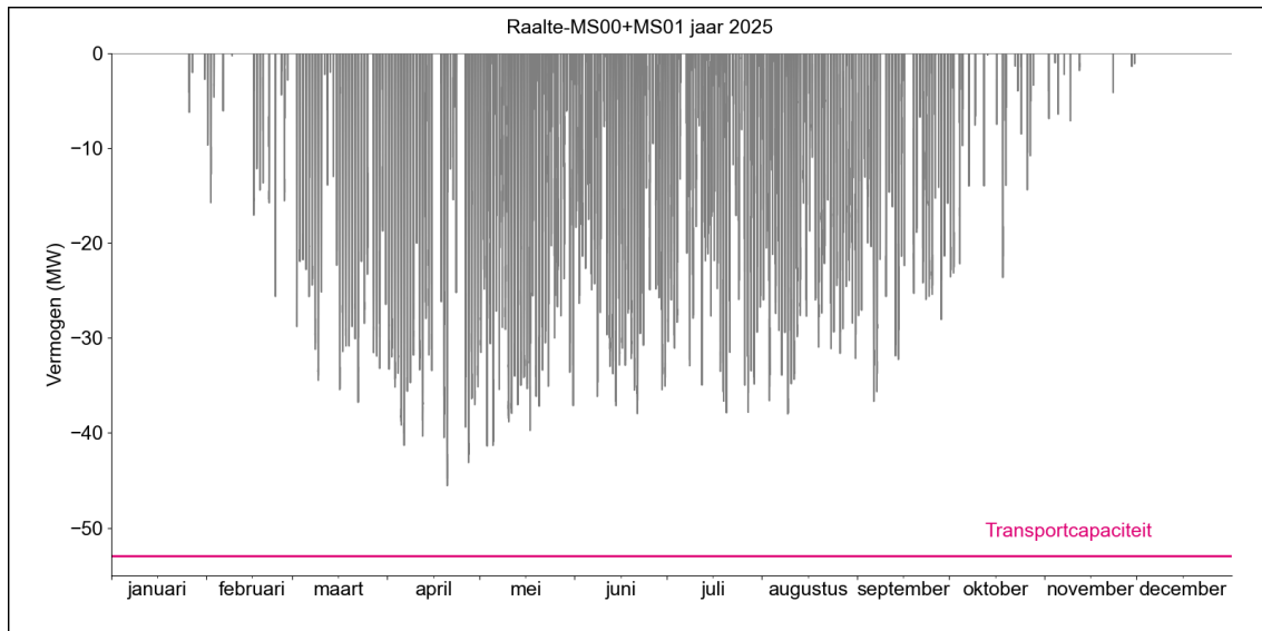
Figuur 2. Gerealiseerde transportbelasting voor invoeding op HS/MS-station Raalte MS00 + MS01 in 2025.
