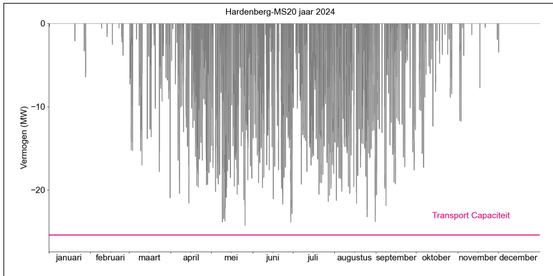
Figuur 2. Gerealiseerde transportbelasting voor invoeding op HS/MS-station Hardenberg MS20 in 2024.
