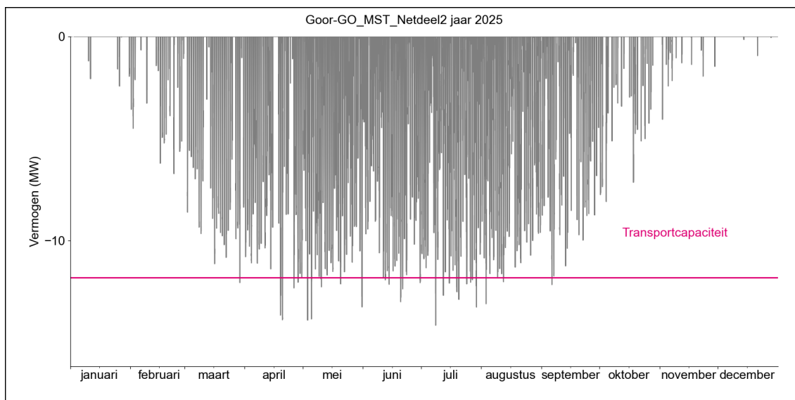
Figuur 2. Gerealiseerde transportbelasting voor invoeding op netdeel Goor GO_MST_Netdeel2 in 2025.
