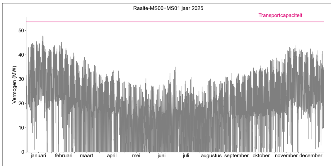
Figuur 2. Gerealiseerde transportbelasting voor afname op HS/MS-station Raalte MS00 + MS01 in 2025.
