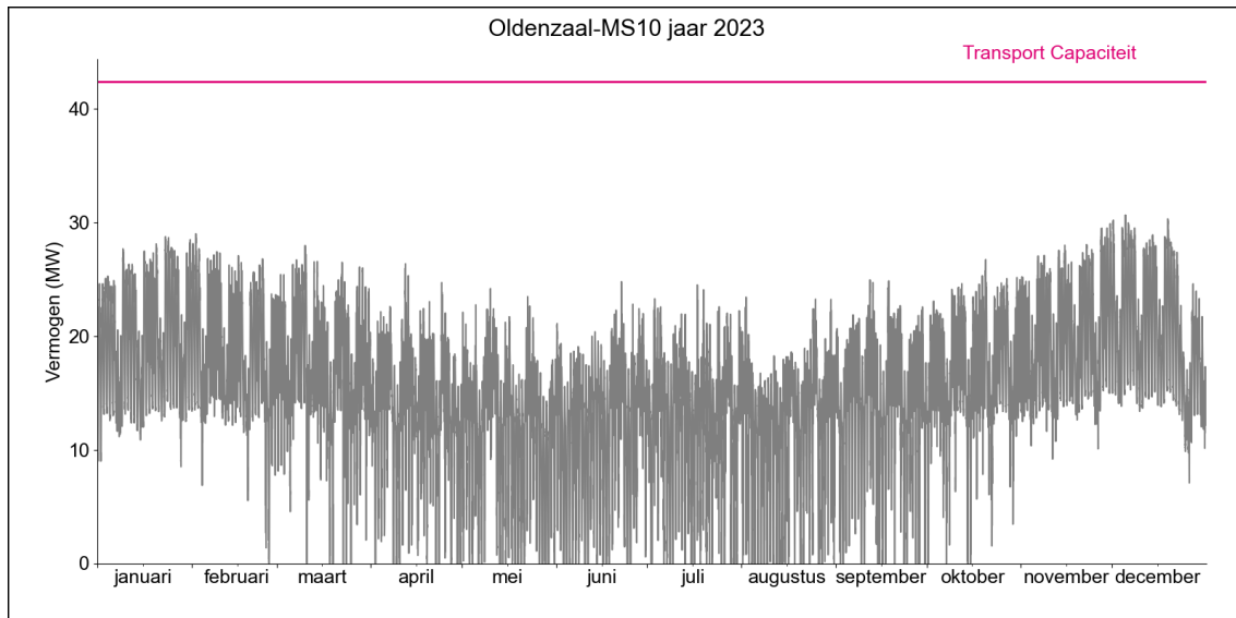
Figuur 2. Gerealiseerde transportbelasting voor afname op HS/MS-station Oldenzaal MS10 in 2023.
