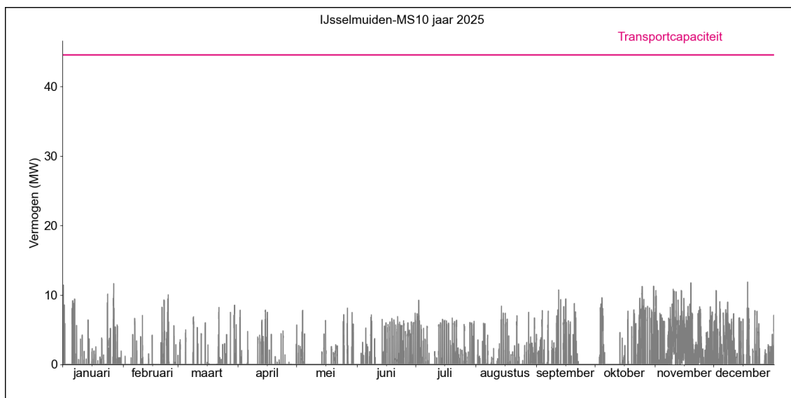
Figuur 2. Gerealiseerde transportbelasting voor afname op HS/MS-station IJsselmuiden MS10 in 2025.
