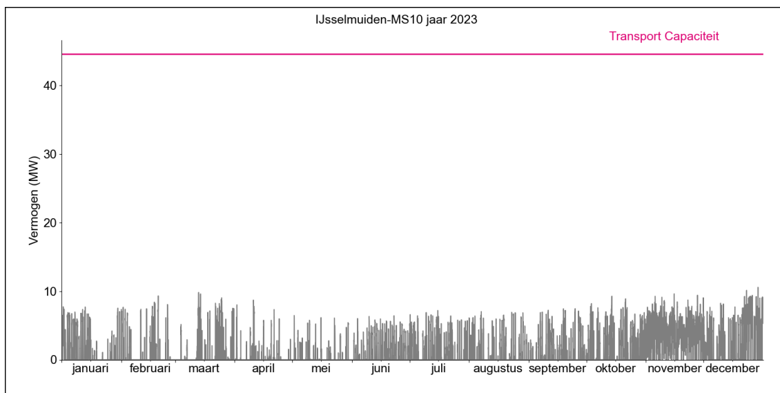
Figuur 2. Gerealiseerde transportbelasting voor afname op HS/MS-station IJsselmuiden MS10 in 2023.
