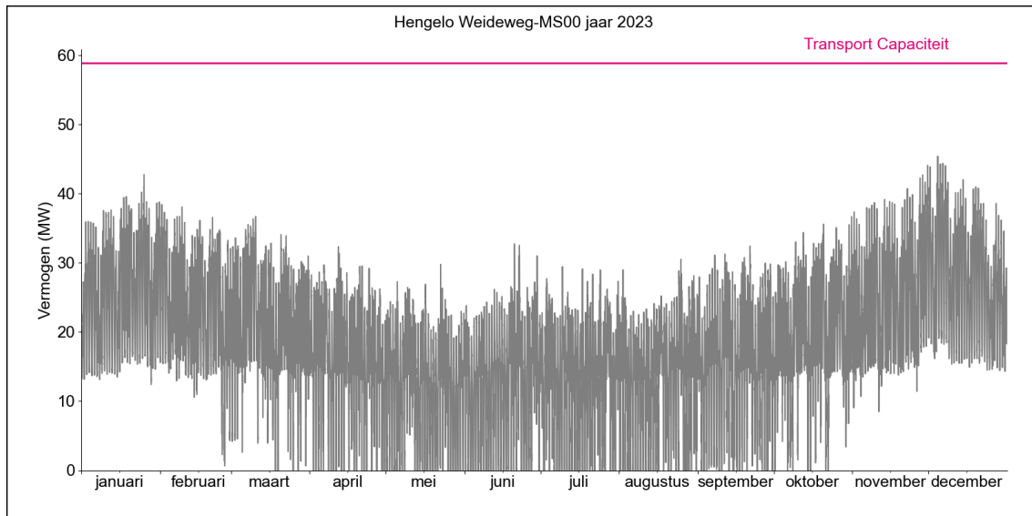
Figuur 2. Gerealiseerde transportbelasting voor afname op HS/MS-station Hengelo Weideweg MS00 in 2023.
