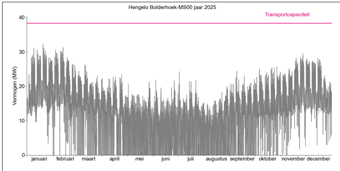
Figuur 2. Gerealiseerde transportbelasting voor afname op HS/MS-station Hengelo Bolderhoek MS00 in 2025.
