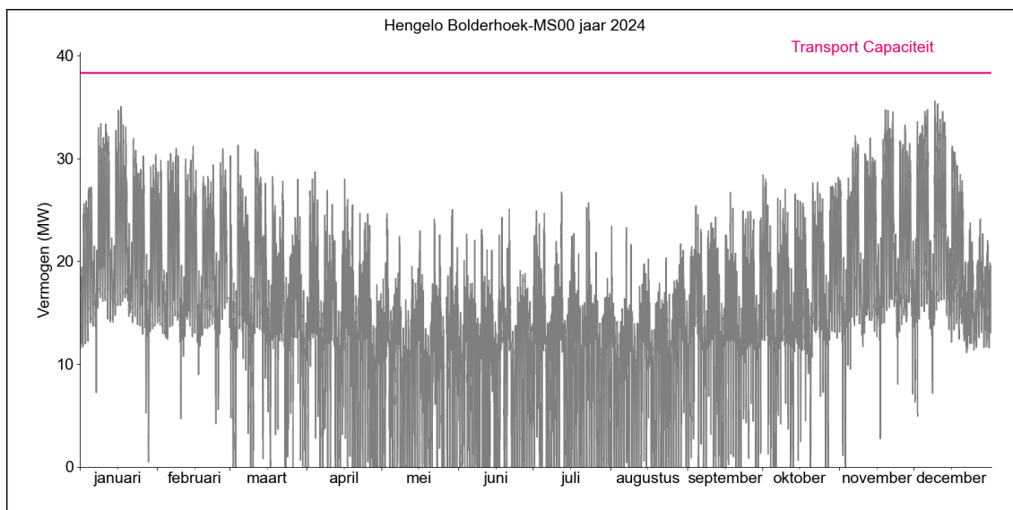
Figuur 2. Gerealiseerde transportbelasting voor afname op HS/MS-station Hengelo Bolderhoek MS00 in 2024.
