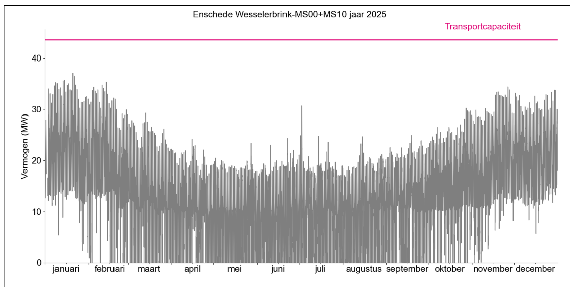
Figuur 2. Gerealiseerde transportbelasting voor afname op HS/MS-station Enschede Wesselerbrink MS00 + MS10 in 2025.
