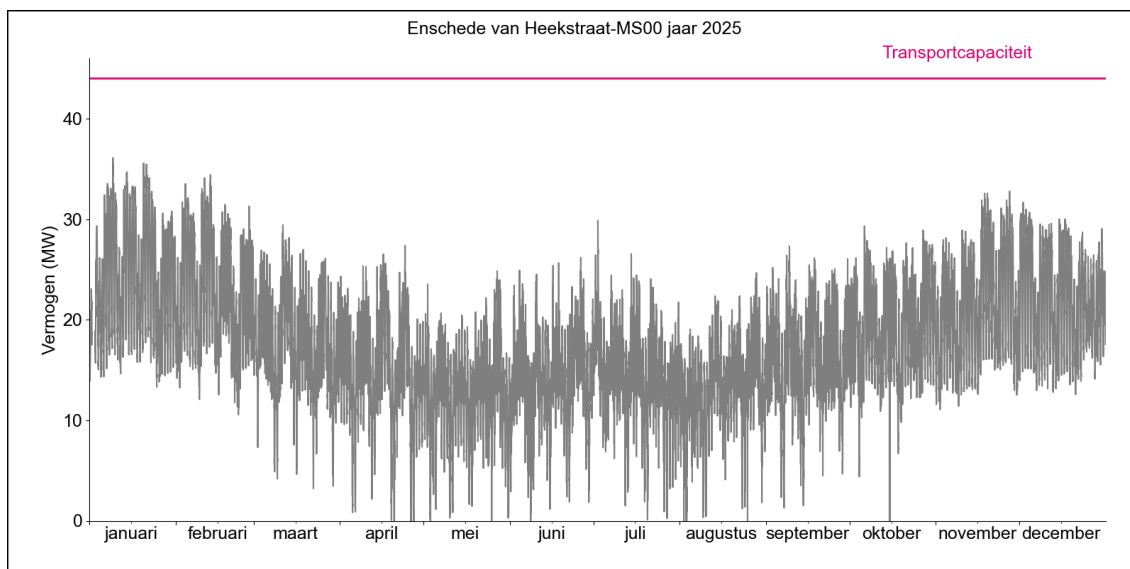
Figuur 2. Gerealiseerde transportbelasting voor afname op HS/MS-station Enschede van Heekstraat MS00 in 2025.
