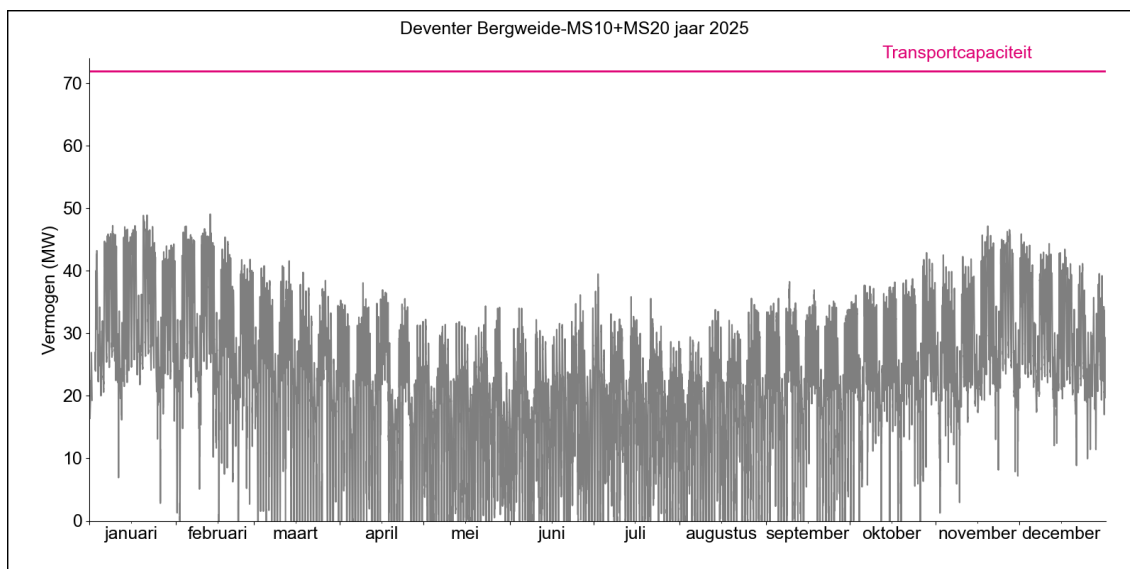
Figuur 2. Gerealiseerde transportbelasting voor afname op HS/MS-station Deventer Bergweide MS00 + MS01 + MS10 in 2025.
