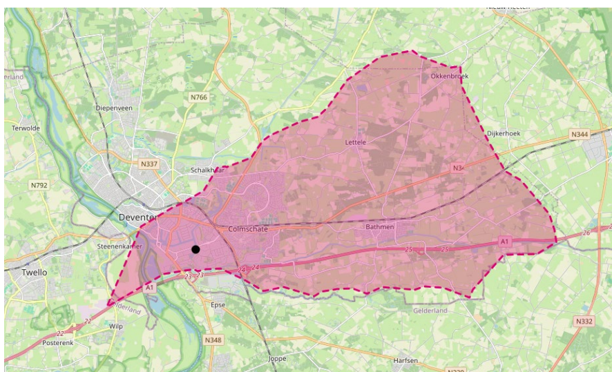
Figuur 1. Geografische indicatie van het voorzieningsgebied van HS/MS-station Deventer Bergweide MS00 + MS01 + MS10.
