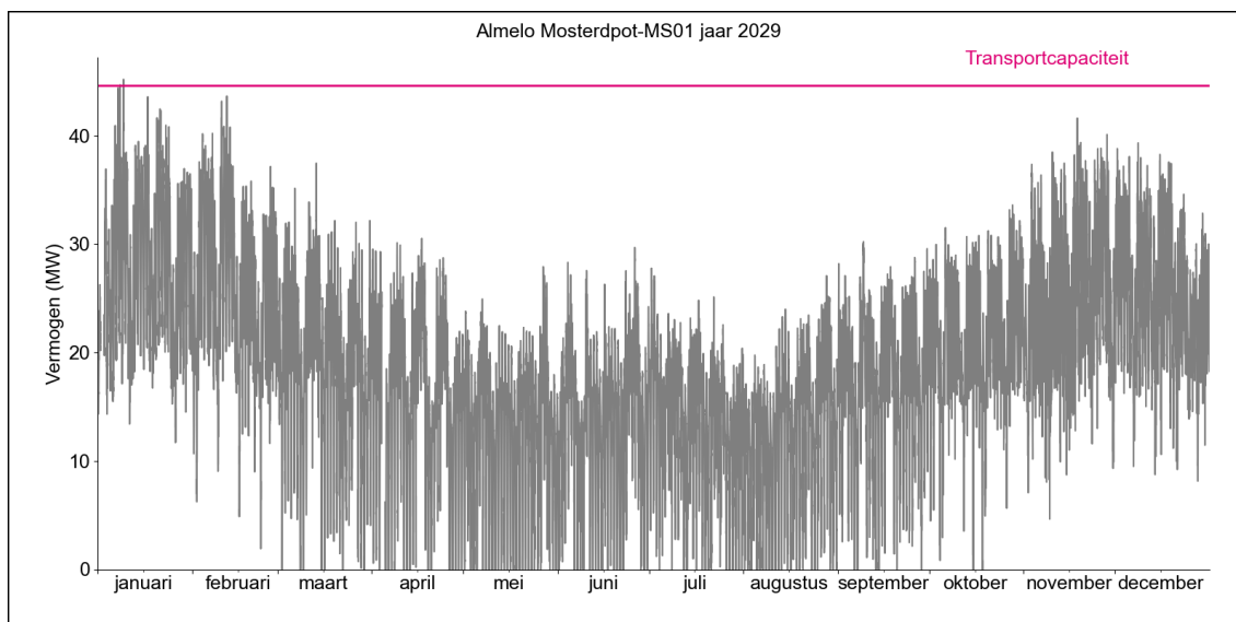
Figuur 2. Prognose van de benodigde transportcapaciteit in 2029.
