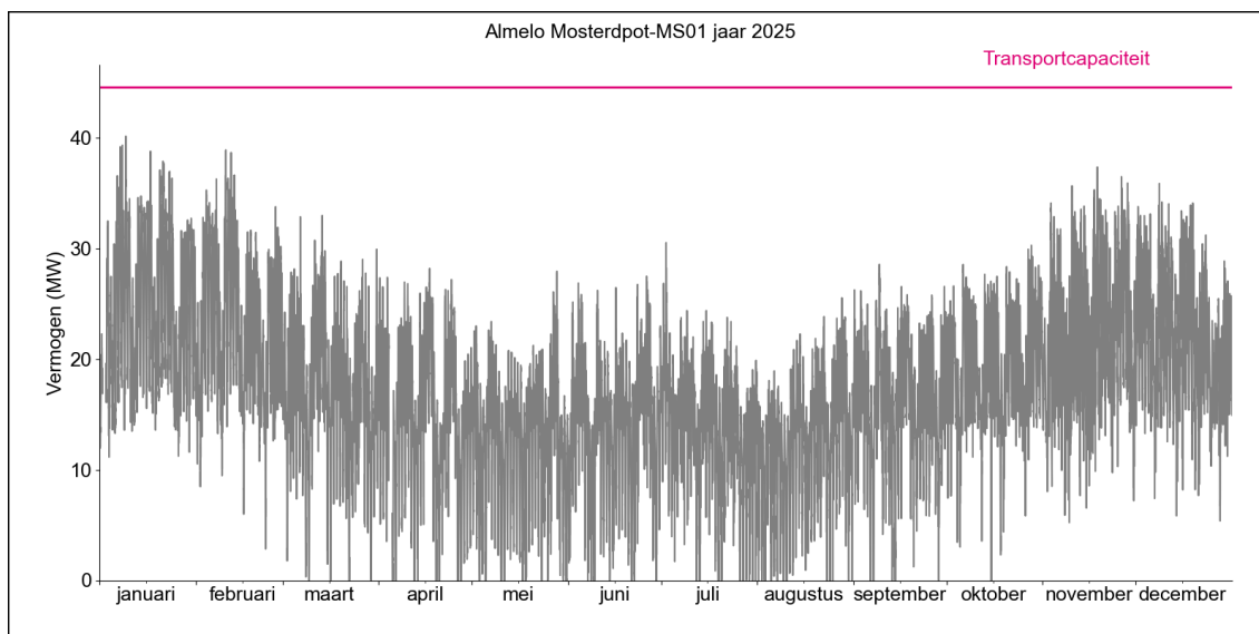
Figuur 1. Gerealiseerde transportbelasting voor afname op HS/MS-station Almelo Mosterdpot MS01 in 2025.
