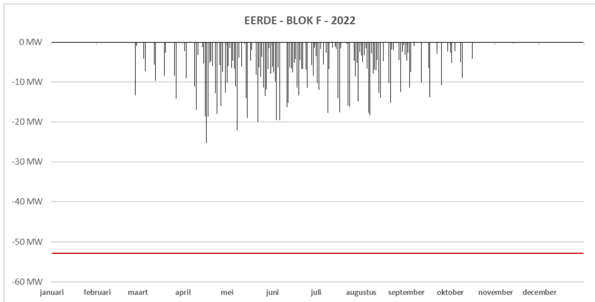
Figuur 2. Gemeten transportbelasting op station Eerde blok F in 2022. Een negatieve waarde representeert invoeding in het hoogspanningsnet. De huidige, aanwezige transportcapaciteit voor invoeding bedraagt 52,8 MW.
