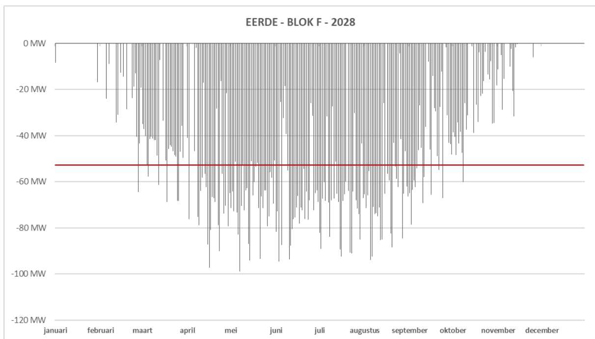
Figuur 3. Verwachte transportbelasting op station Eerde blok F in het laatste jaar van de congestie.
