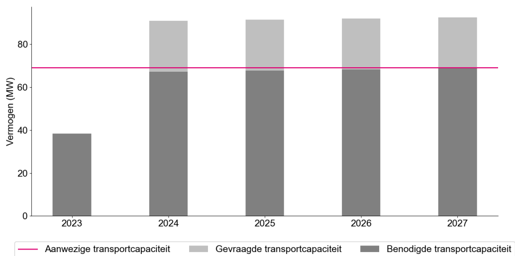
Benodigde en gevraagde transportcapaciteit Afname MDK-Blok B
