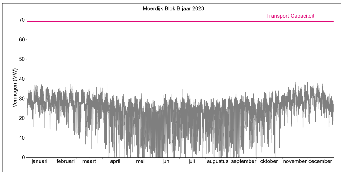
Figuur 2. Gerealiseerde transportbelasting voor afname op HS/MS-station Moerdijk Blok B in 2023.
