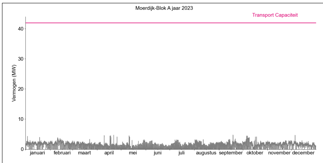
Figuur 2. Gerealiseerde transportbelasting voor afname op HS/MS-station Moerdijk Blok A in 2023.
