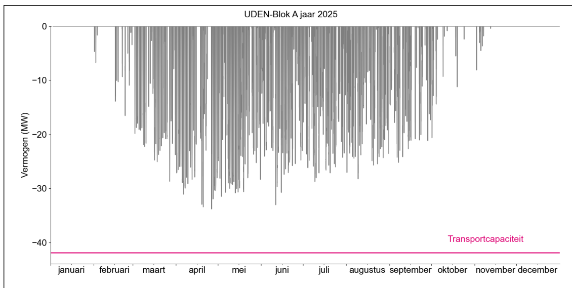
Figuur 2. Gerealiseerde transportbelasting voor invoeding op HS/MS-station Uden Blok A in 2025.
