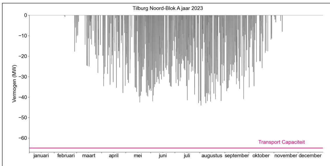
Figuur 2. Gerealiseerde transportbelasting voor invoeding op HS/MS-station Tilburg Noord Blok A in 2023.
