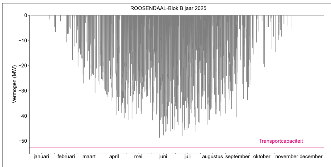
Figuur 2. Gerealiseerde transportbelasting voor invoeding op HS/MS-station Roosendaal Blok B in 2025.
