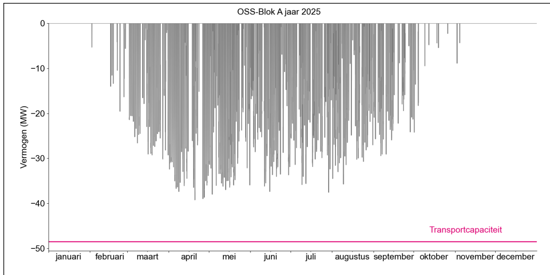
Figuur 2. Gerealiseerde transportbelasting voor invoeding op HS/MS-station Oss Blok A in 2025.
