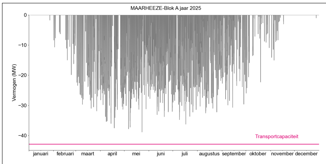
Figuur 2. Gerealiseerde transportbelasting voor invoeding op HS/MS-station Maarheeze Blok A in 2025.
