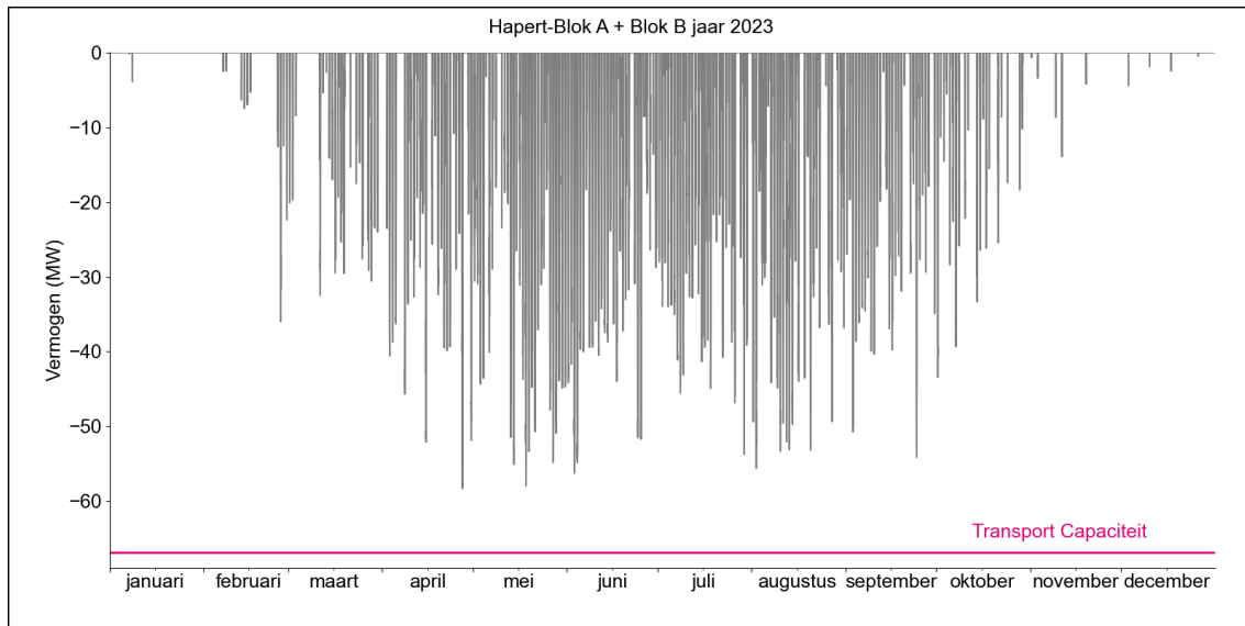
Figuur 2. Gerealiseerde transportbelasting voor invoeding op HS/MS-station Hapert Blok A + Blok B in 2023.
