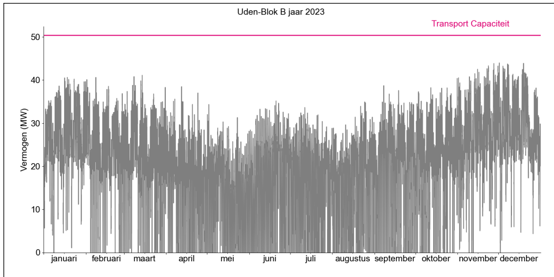
Figuur 2. Gerealiseerde transportbelasting voor afname op HS/MS-station Uden Blok B in 2023.
