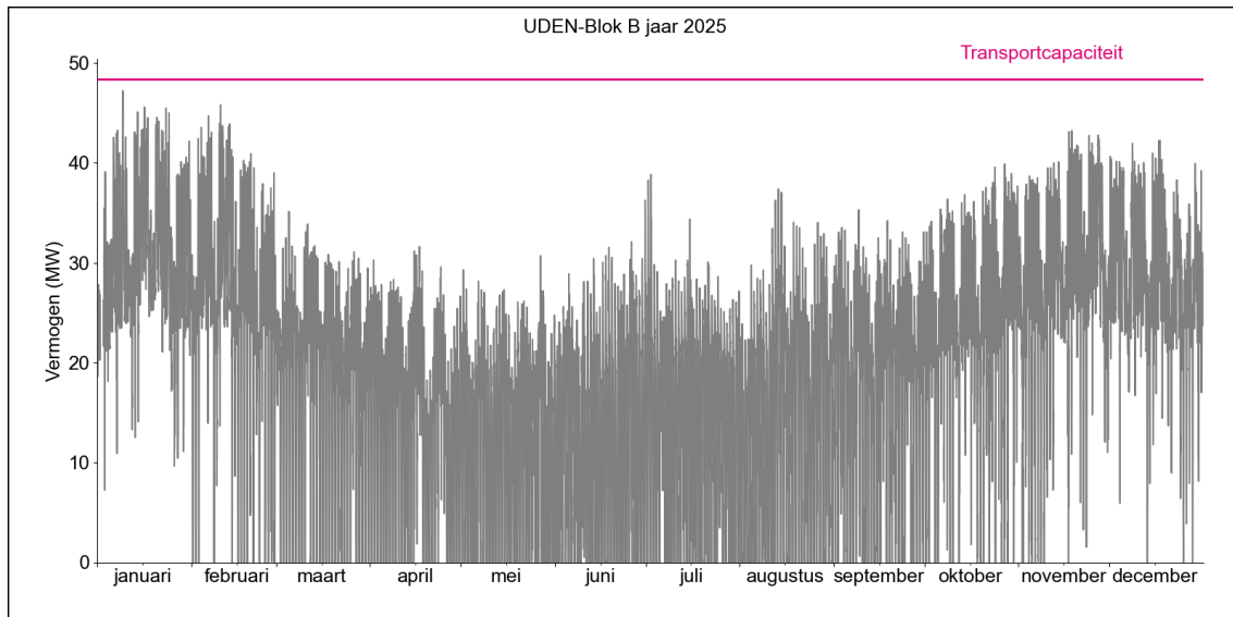
Figuur 2. Gerealiseerde transportbelasting voor afname op HS/MS-station Uden Blok B in 2025.
