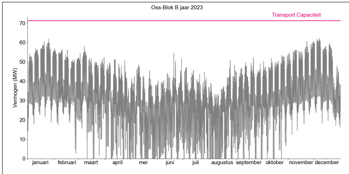
Figuur 2. Gerealiseerde transportbelasting voor afname op HS/MS-station Oss Blok B in 2023.
