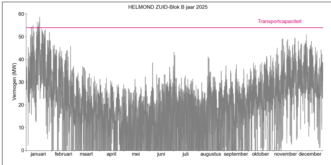
Figuur 2. Gerealiseerde transportbelasting voor afname op HS/MS-station Helmond Zuid Blok B in 2025.
