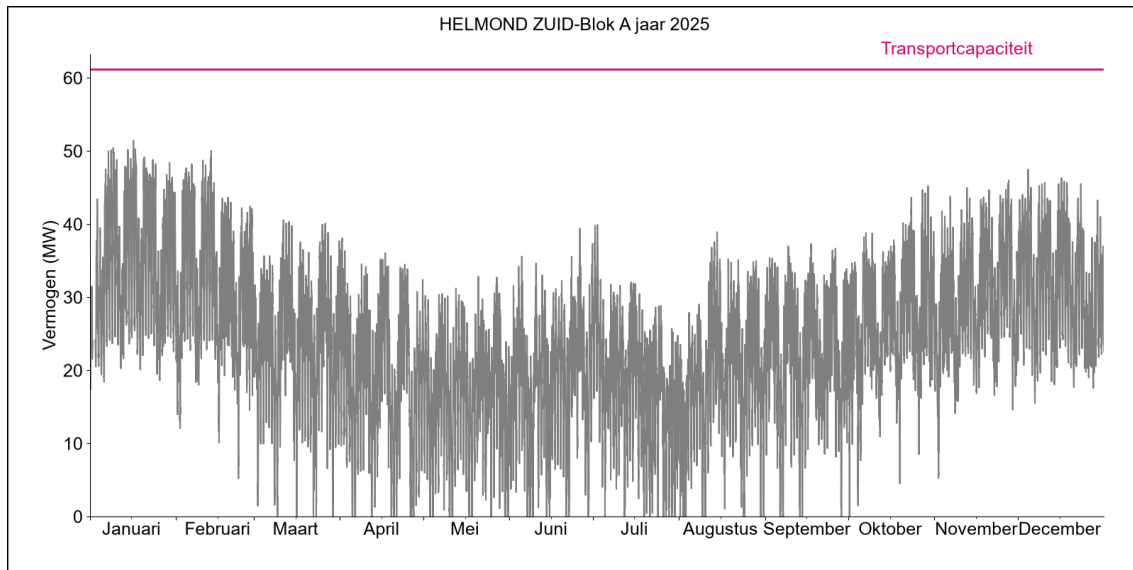
Figuur 2. Gerealiseerde transportbelasting voor afname op HS/MS-station Helmond Zuid Blok A in 2025.
