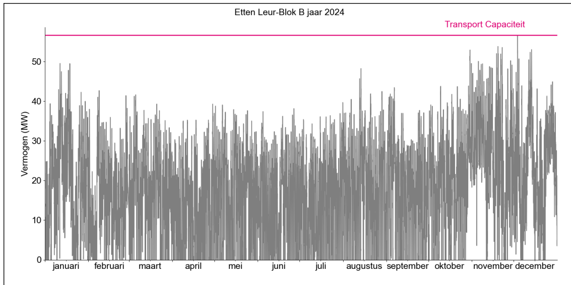
Figuur 2. Gerealiseerde transportbelasting voor afname op HS/MS-station Etten Leur Blok B in 2024.
