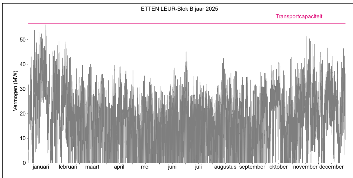
Figuur 2. Gerealiseerde transportbelasting voor afname op HS/MS-station Etten Leur Blok B in 2025.
