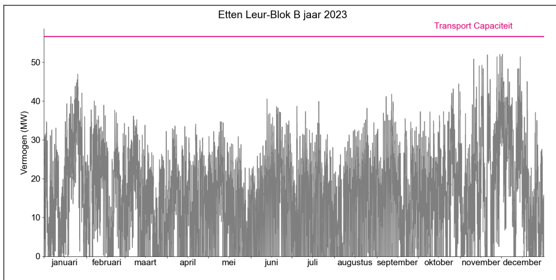
Figuur 2. Gerealiseerde transportbelasting voor afname op HS/MS-station Etten Leur Blok B in 2023.
