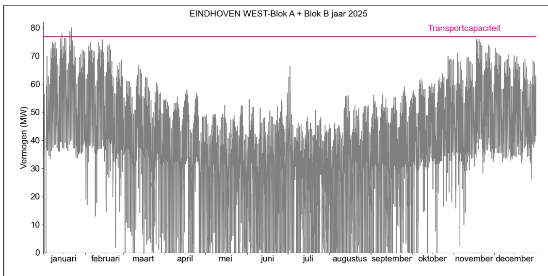
Figuur 2. Gerealiseerde transportbelasting voor afname op HS/MS-station Eindhoven West Blok A + Blok B in 2025.
