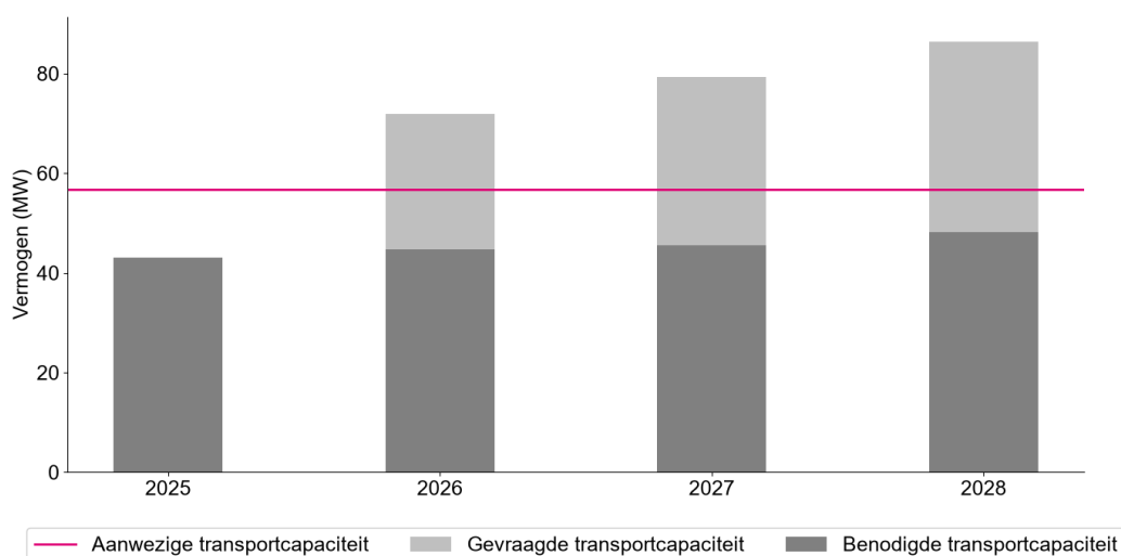
Figuur 4. Prognose van de benodigde en gevraagde transportcapaciteit per jaar.
