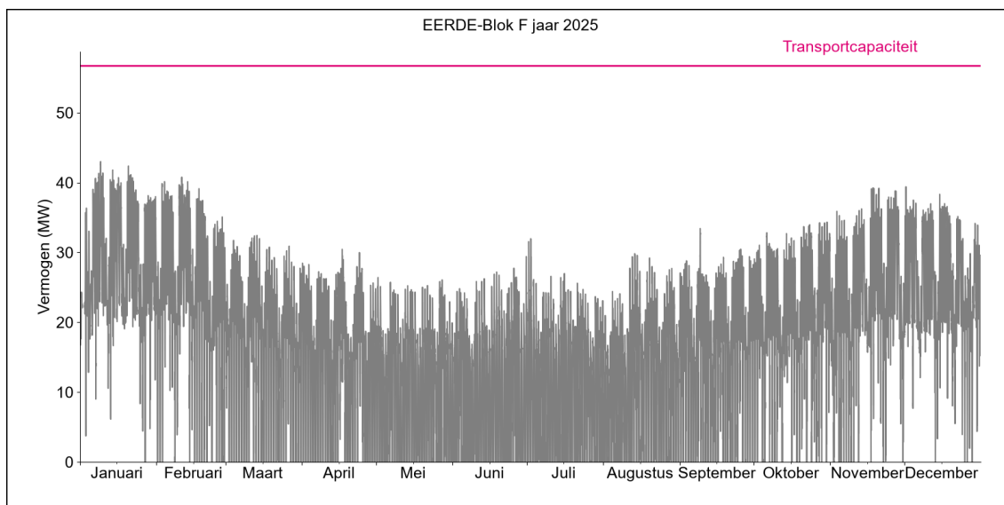
Figuur 2. Gerealiseerde transportbelasting voor afname op HS/MS-station Eerde Blok F in 2025.
