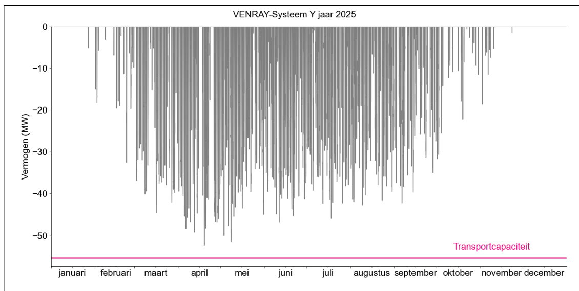
Figuur 2. Gerealiseerde transportbelasting voor invoeding op HS/MS-station Venray Systeem Y in 2025.
