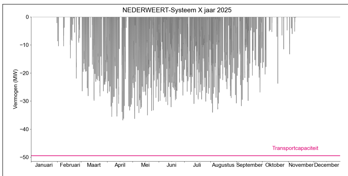
Figuur 2. Gerealiseerde transportbelasting voor invoeding op HS/MS-station Nederweert Systeem X in 2025.
