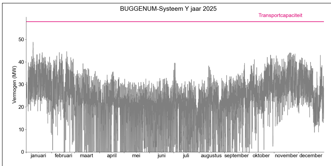
Figuur 2. Gerealiseerde transportbelasting voor afname op HS/MS-station Buggenum Systeem Y in 2025.
