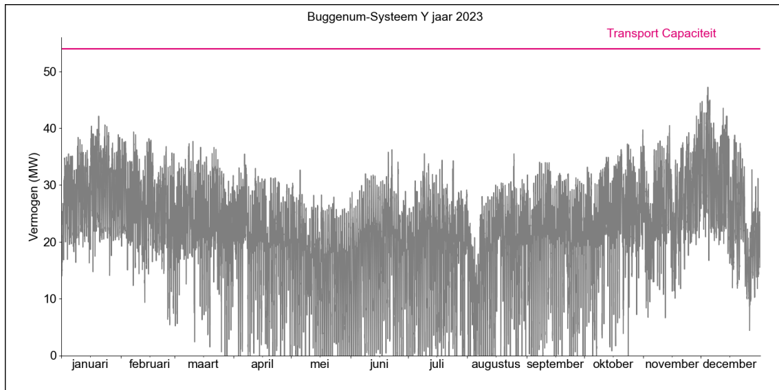
Figuur 2. Gerealiseerde transportbelasting voor afname op HS/MS-station Buggenum Systeem Y in 2023.
