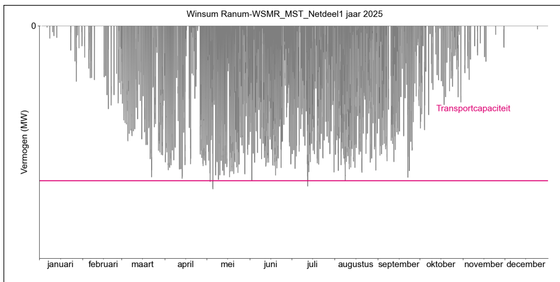
Figuur 2. Gerealiseerde transportbelasting voor invoeding op netdeel Winsum Ranum WSMR_MST_Netdeel1 in 2025.
